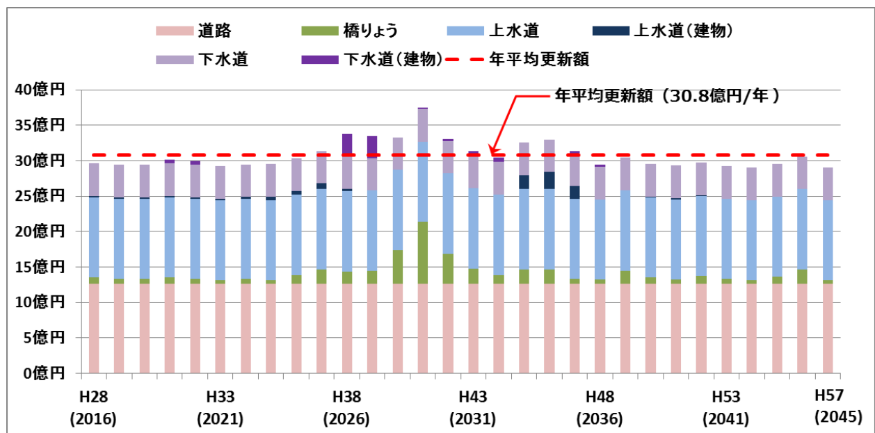
図 インフラ施設と上下水道関連建物の将来更新費
