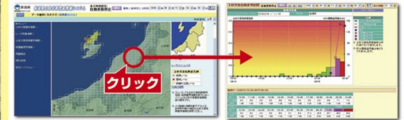
土砂災害危険度メッシュ図
