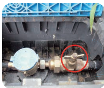
▲メーターボックス内にある止水栓
